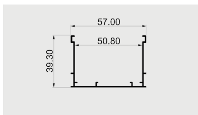
Profilo per INCASSO 50 (disponibile col. semilucido RAL 9010/RAL 1013/RAL 8017)
