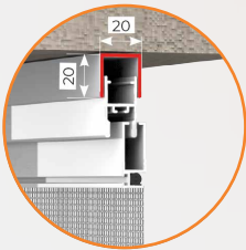
STANDARD - Optional Kit compensazione
