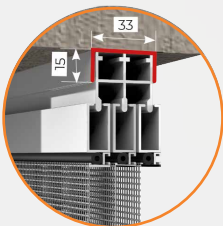
OPTIONAL 3 ANTE Kit compensazione
