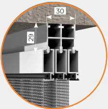
STANDARD Scorrevole 3 ante
