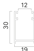
Guida alluminio 30x19 mm con spazzolino 4,8x4
