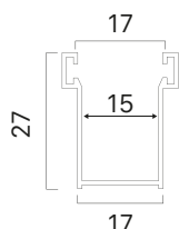
Guida alluminio 27x17 mm con spazzolino 4,8x6
