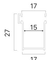
Guida alluminio 27x17 mm con spazzolino 4,8x3
