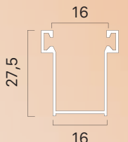
Guida alluminio 28x16 mm con spazzolino 4,8x4
