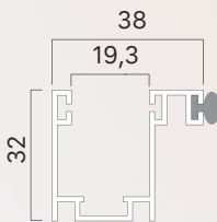
Pretelaio 32x38 mm con spazzolino 4,8x6
