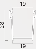
Guida alluminio 28x19 mm con spazzolino 4,8x4
