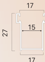
Guida alluminio 27x17 mm con spazzolino 4,8x4
