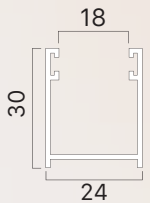
Guida alluminio 30x24 mm con spazzolino 4,8x5
