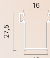
Guida alluminio 28x16 mm con spazzolino 4,8x6
