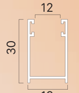
Guida alluminio 30x19 mm con spazzolino 4,8x4
