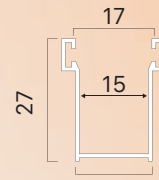
Guida alluminio 27x17 mm con spazzolino 4,8x4
