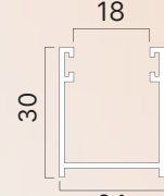
Guida alluminio 30x24 mm con spazzolino 4,8x5
