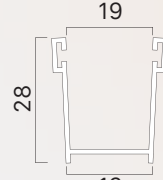
Guida alluminio 28x19 mm con spazzolino 4,8x4
