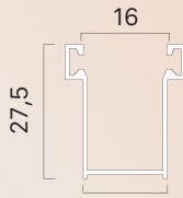
Guida alluminio 28x16 mm con spazzolino 4,8x6
