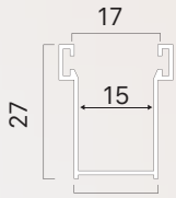
Guida alluminio 27x17 mm con spazzolino 4,8x6
