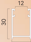
Guida alluminio 30x19 mm con spazzolino 4,8x4
