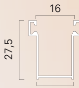
Guida alluminio 28x16 mm con spazzolino 4,8x6
